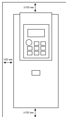
Рис. 3.1 – Требования к минимальным воздушным зазорам
