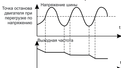
Рис. 6.25 Защита при превышении напряжения
