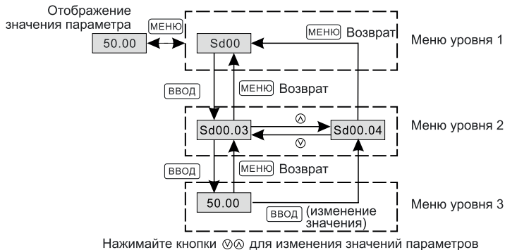
Рис 6.1 Схема настройки параметров меню
